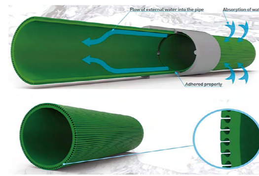
ドレインパイプ。専用ソケットにより、表面から吸い上げた水はパイプの中へ流れる
