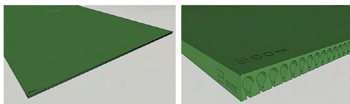
ドレインベルト 幅200mm×厚さ2mm
