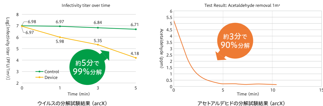
ウイルスの分解試験結果 (arcX)
